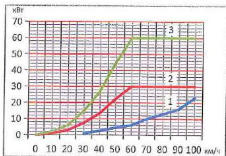
Рис. 3. Характеристики ветрогенераторов: 1 — 40 кВт, 700 об/мин (TGЕТ770-І-Н-40KW-700R); 2 — 30 кВт, 300 об/мин (TGЕТ770-І-30KW-300R); 3 — 60 кВт, 300 об/мин (TGЕТ900-І-60KW-300R)
