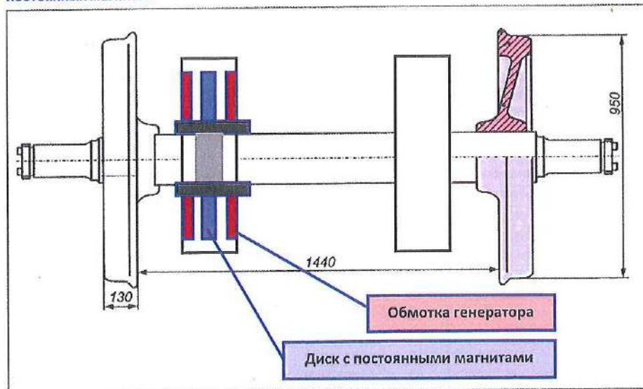
Рис. 6. Схема установки тормозного генератора на колесную пару
