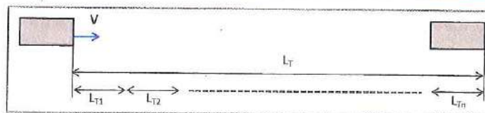
Рис. 2. Схема торможения вагона на участке
